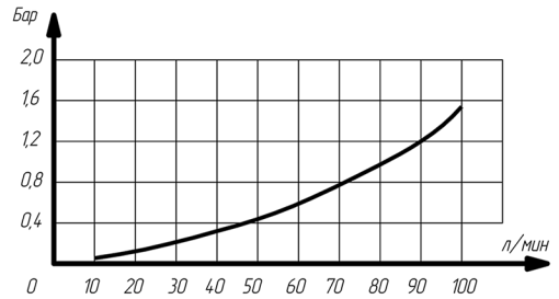
График падения давления
