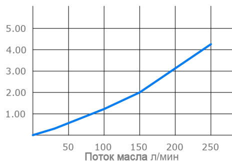
Перепад давления
