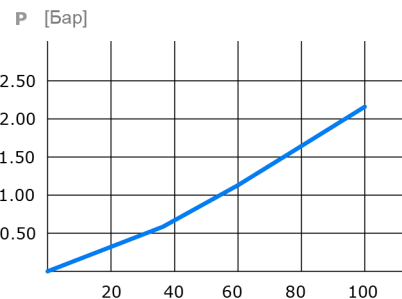
Перепад давления
