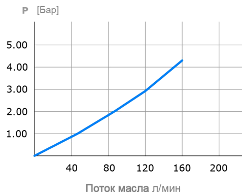
Перепад давления
